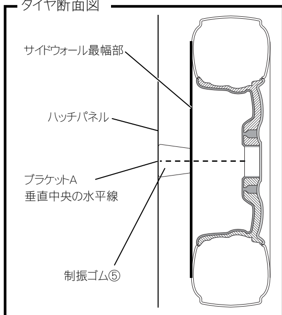
タイヤ断面図
