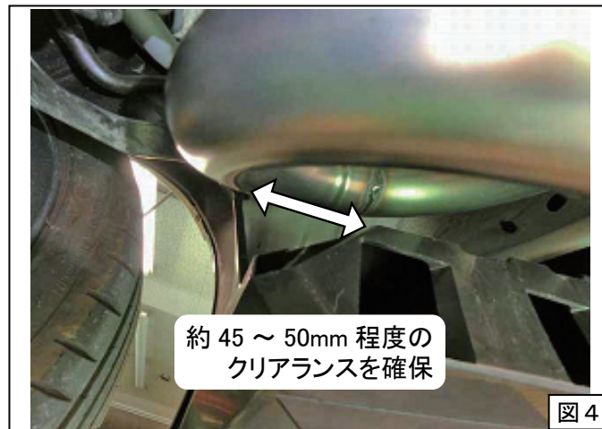
図 4. 加工後のリアバンパーサイドカバーと メインマフラーのクリアランス
