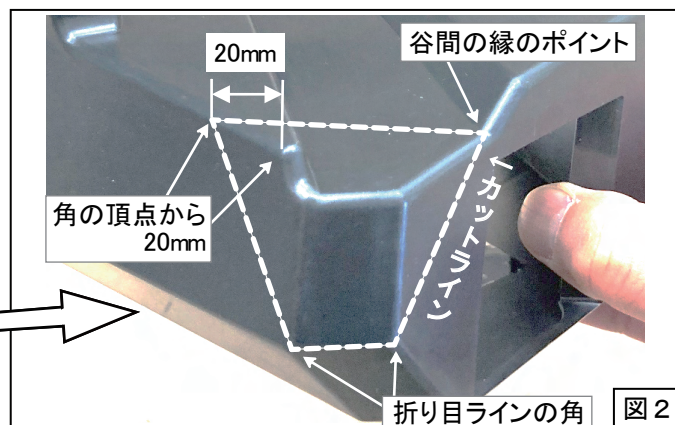
図2. 加工部詳細とカットライン決めのポイント
