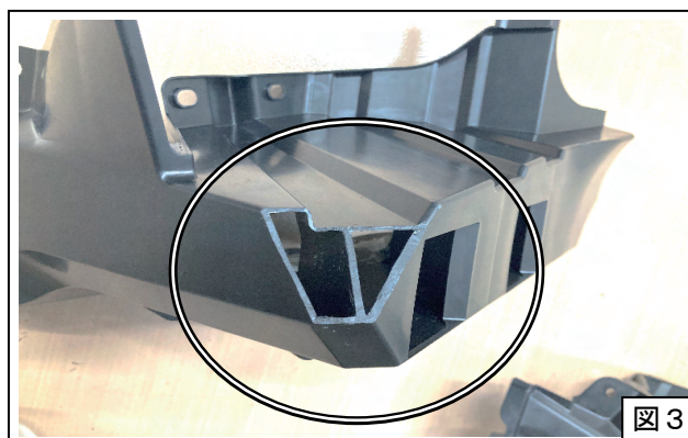
図3. 加工後のリアバンパーサイドカバー
